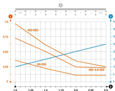
Belastningsdiagram trådstege GR-Magic typ GRM 55
