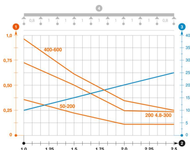
Belastningsdiagram trådstege typ GRM 55 VA
