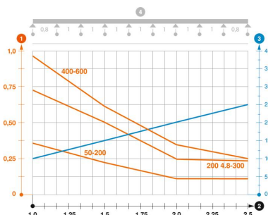
Belastningsdiagram trådstege GR-Magic typ GRM 55
