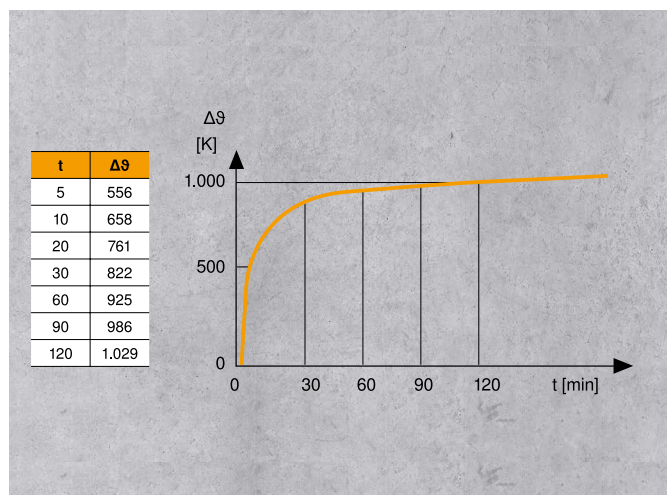
Temperaturtidskurva enligt SS EN 1363-1.
