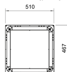
Dimension ingjutningslåda
